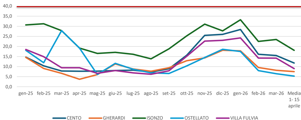
Figura 1.4 – Dati sulla qualità dell'aria, NO 2 nelle stazioni della rete regionale della provincia di Ferrara, dal 01/01/2025 al 01/04/2026, valori medi µg/m 3
