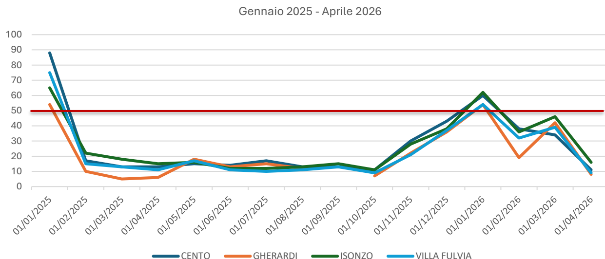
Figura 1.2 – Dati sulla qualità dell'aria, PM10 nelle stazioni della rete regionale della provincia di Ferrara, dal 01/01/2025 al 01/04/2026, valori medi \mu\text{g}/\text{m}^3
