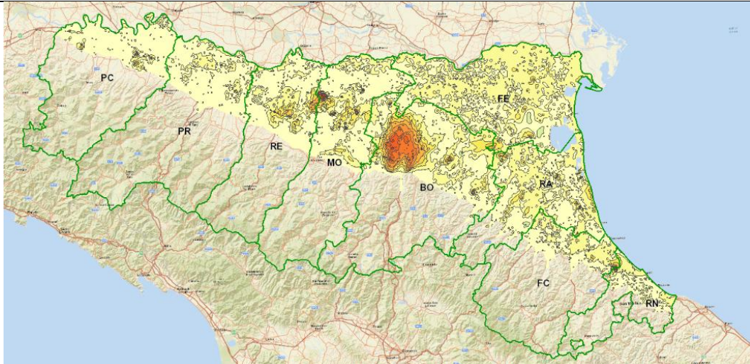
Figura 1.6 - Subsidenza in regione, dati 2021
