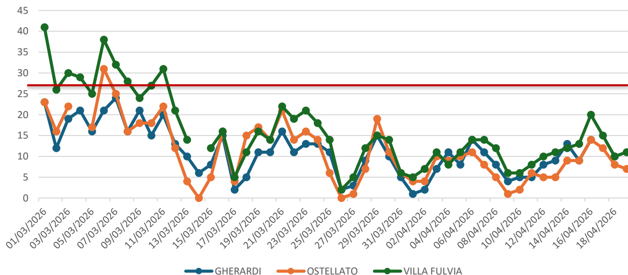
Figura 1.3 – Dati sulla qualità dell'aria, PM2,5 nelle stazioni della rete regionale della provincia di Ferrara, dal 01/03/2026 al 20/04/2026, dati giornalieri \mu\text{g}/\text{m}^3
