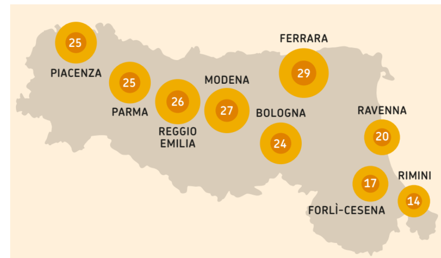
Numero di giorni di disagio bioclimatico nei principali centri urbani dell'Emilia-Romagna, 2025
