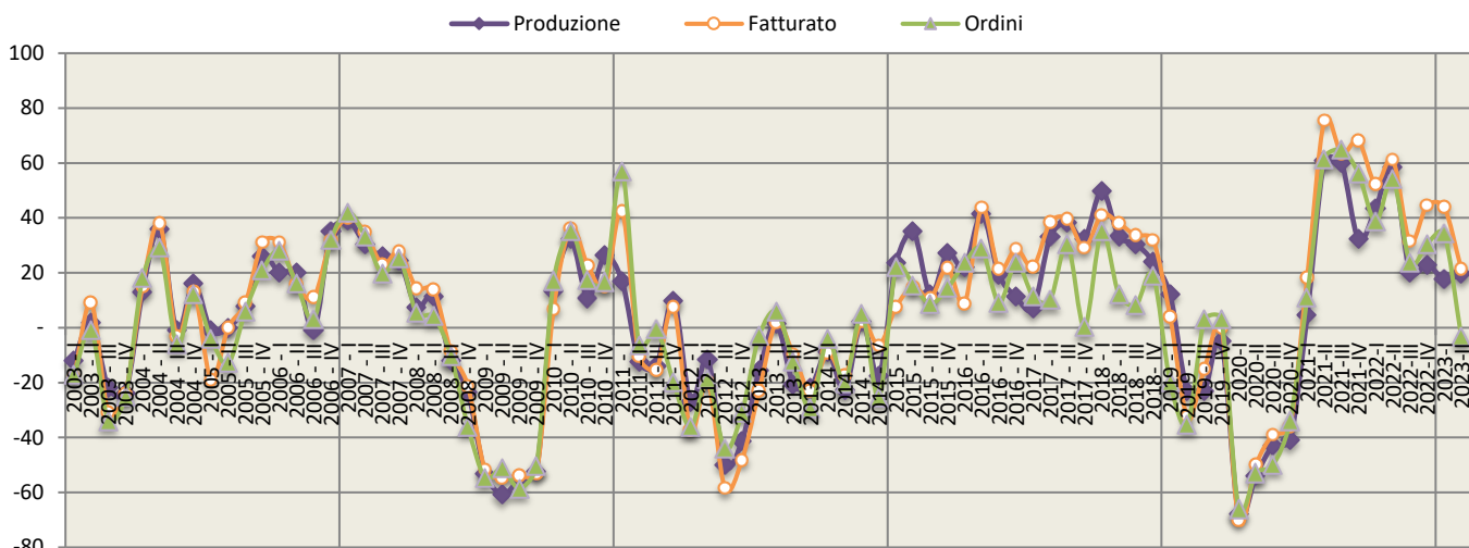
Fig.3 - Indagine congiunturale, Industria in senso stretto, Rimini, saldo trimestre in corso su trimestre anno precedente, 2003-2023 (2°trimestre)
