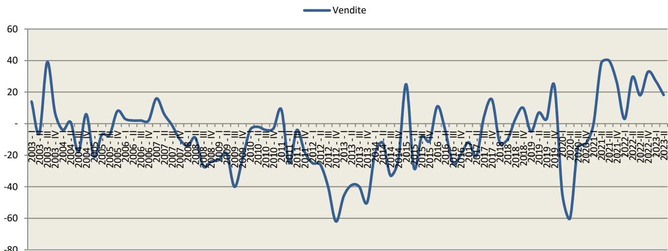
Fig.4 - Indagine congiunturale, Commercio al dettaglio, Rimini, saldo trimestre in corso su trimestre anno precedente, 2003-2023 (2°trimestre)
