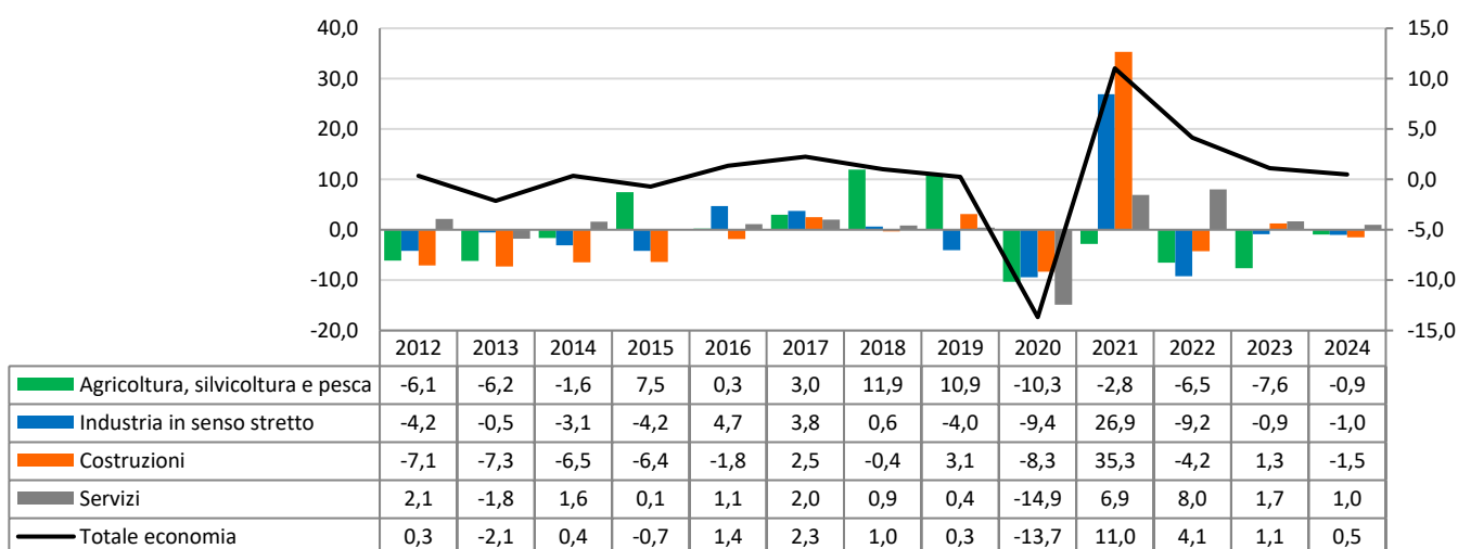
Fig.24 - Andamento delle unità di lavoro totali per settori (Variazione percentuale su anno precedente)
