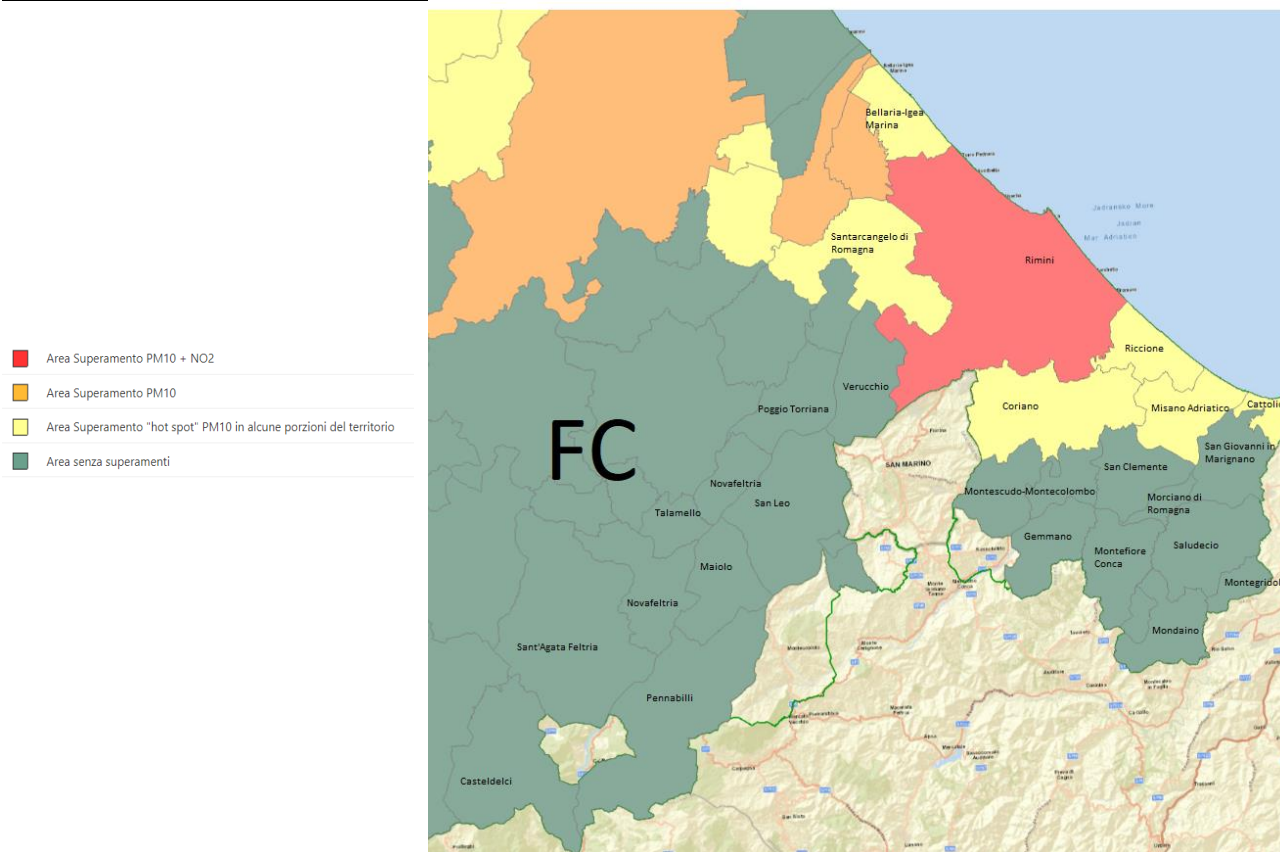
Figura 5.7 - Aree di superamento dei valori limite di PM_{10} E NO_2 – All.1 DRG 26/03/2012 n.362
