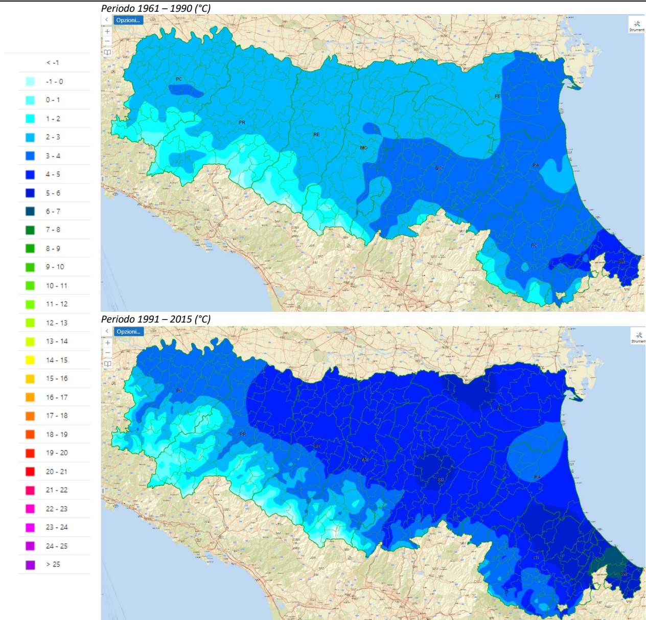
Figura 5.5 - Temperatura media invernale
