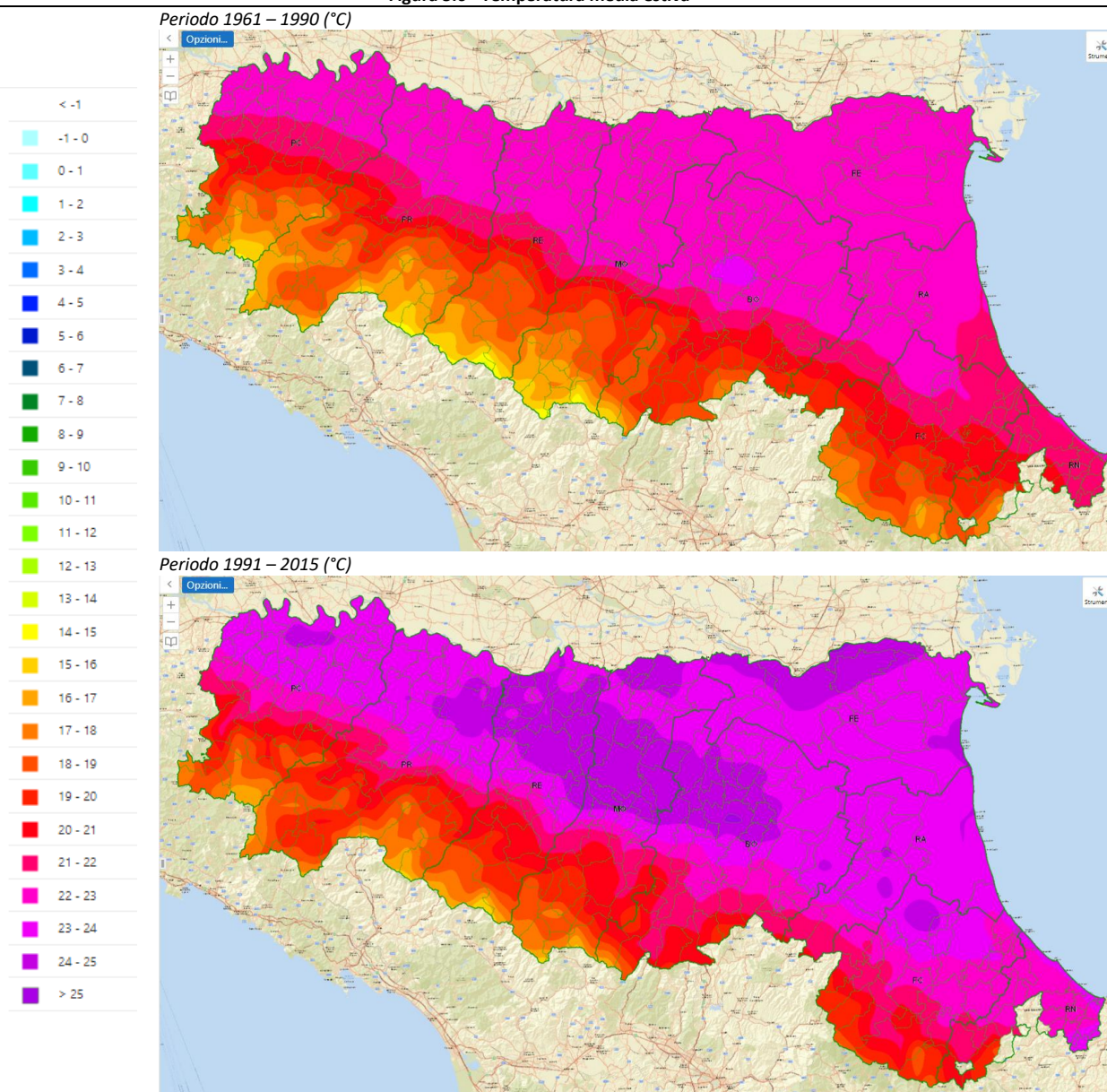
Figura 5.6 - Temperatura media estiva
