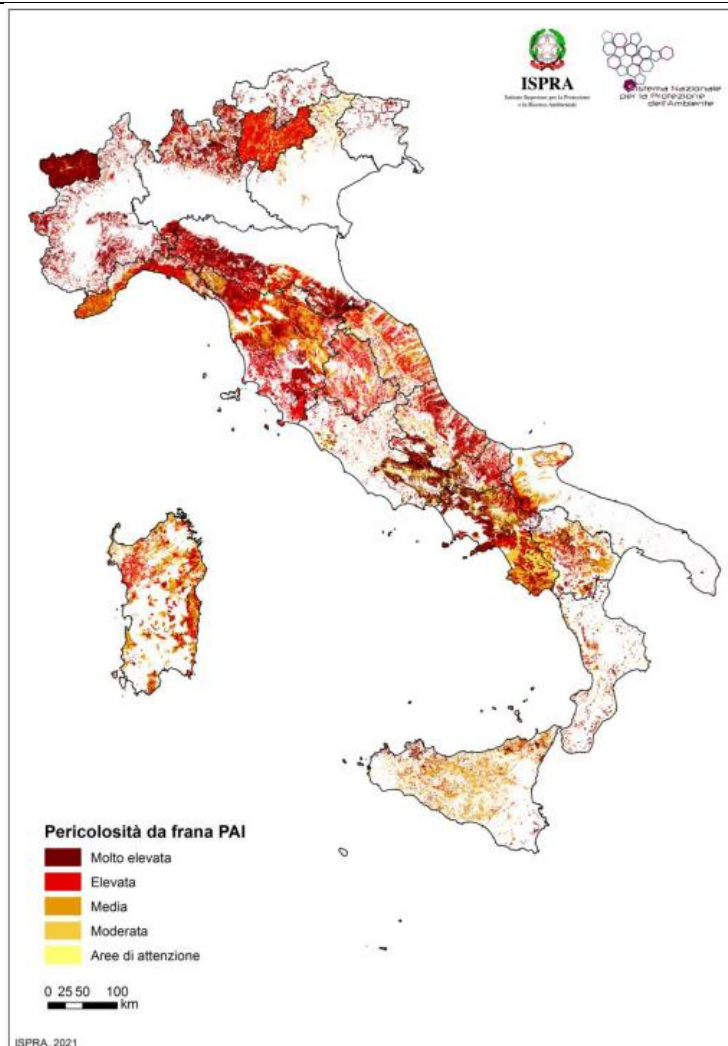
Figura 5.2 – Aree di pericolosità da frana PAI – Mosaicatura 2020-2021
